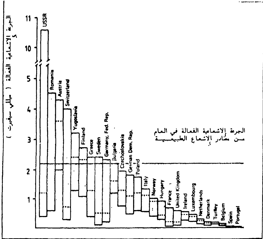
الشكل (٥) مدى توزع الجيرة الإشعاعية الفعالة الناجمة عن حدث تشيرنوبيل ( احتسب من معطيات لجنة الأمم المتحدة العلمية حول آثار الإشعاع 1990 , UNSCEAR )
